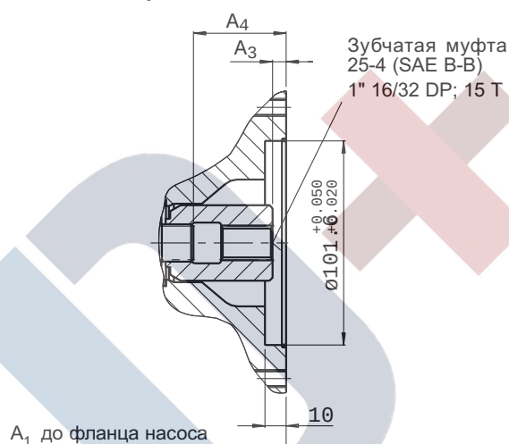
Разрез А - В
