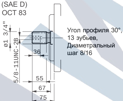
Вид W
