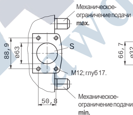
Вид W
