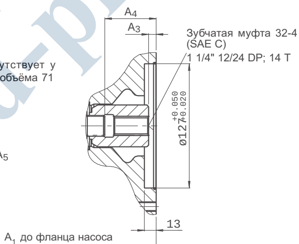
Разрез А - В
