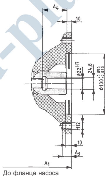
Разрез A - B
